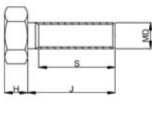
六角头螺栓
