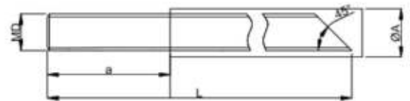
直杆螺栓
