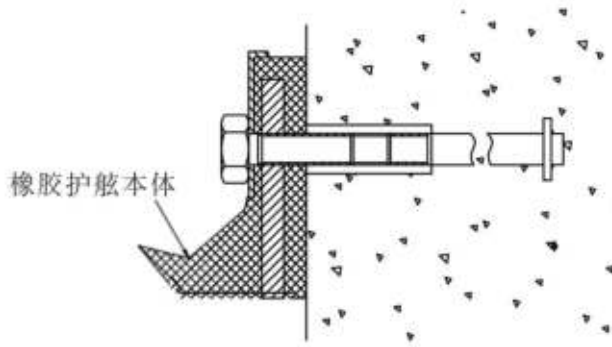
六角头螺栓
